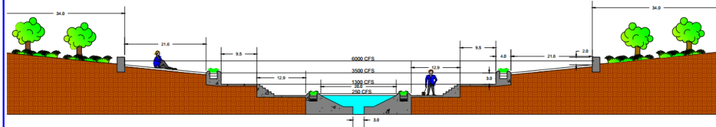
SECTION D-D
